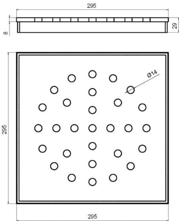
PÖK 8 mm neliökansi mosaiikkibetonille
