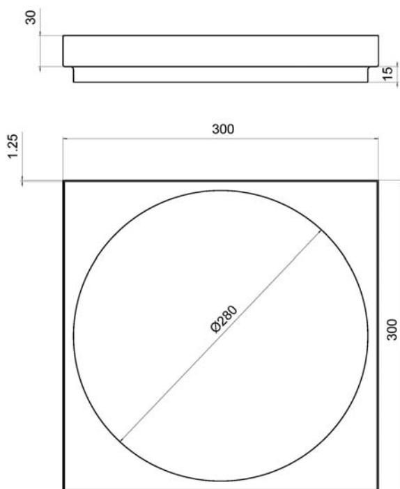
PÖK laattakehys 300 x 300 x 30 mm, sovitussosa 15 mm
