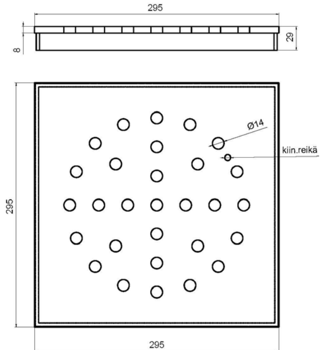
PÖK 8 mm neliökansi mosaiikkibetonille ruuvikiinnityksellä
