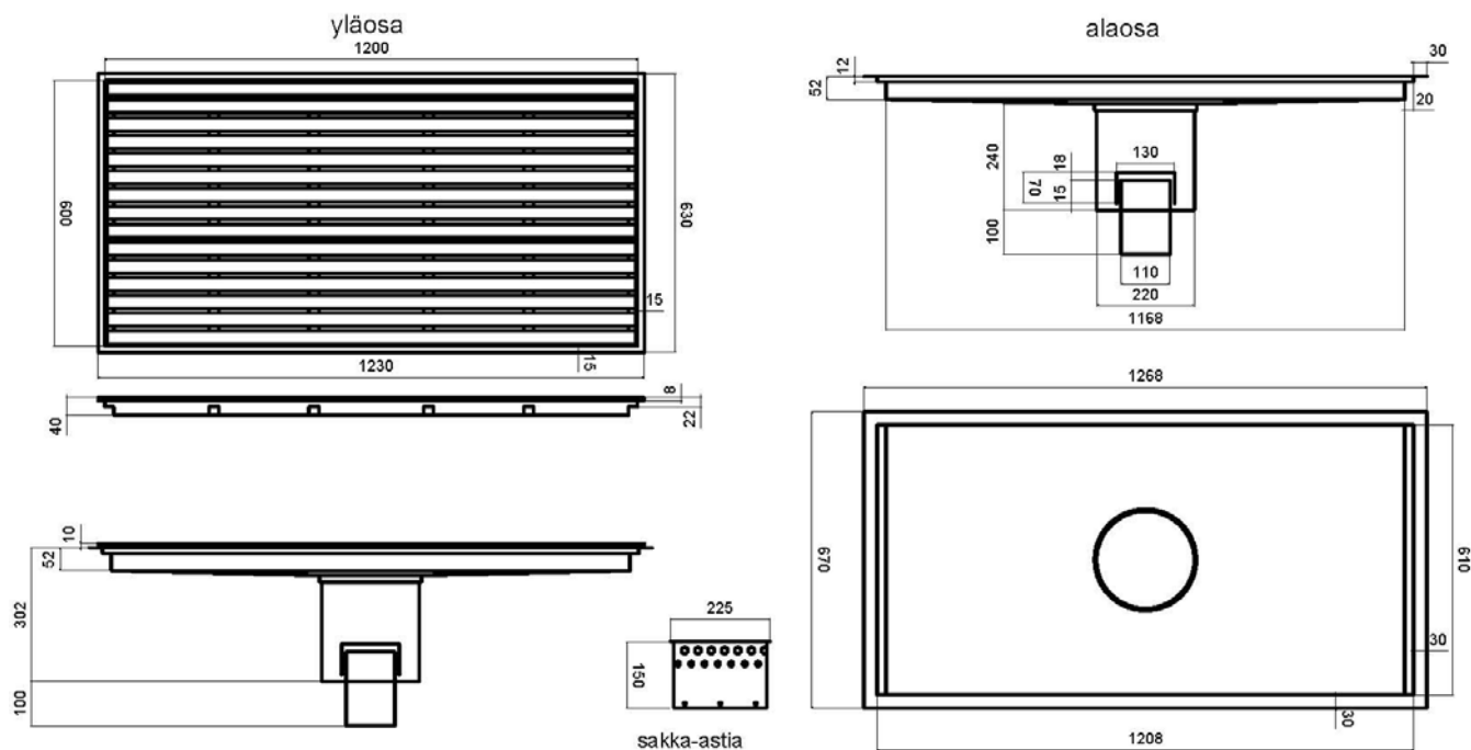
Leveäselkäinen säleritilä
