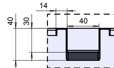
DET1 1:2
