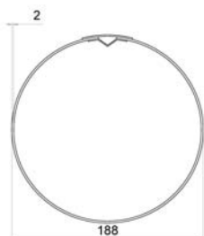
Kiristyskehä kaivokappaleelle
